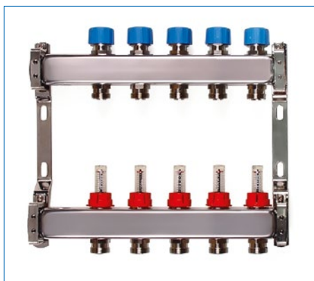
VA-FBif mit Durchflussmengenmesser
